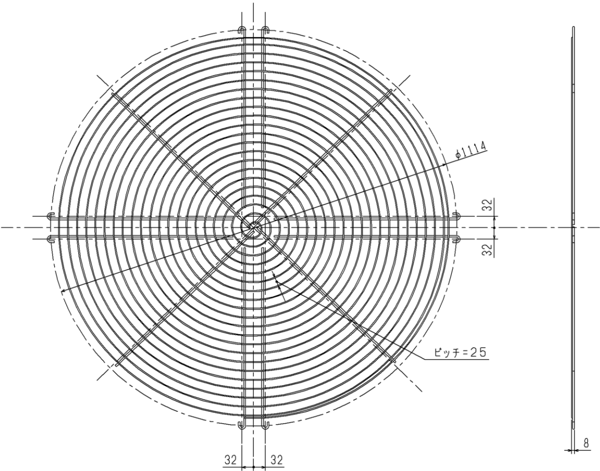
■外形寸法図
