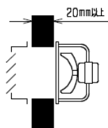
図1 羽根が据付面から出ない場合
