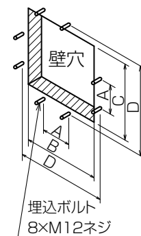
変化寸法表 単位(mm)
